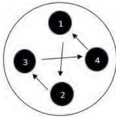
4 Lug Tightening
